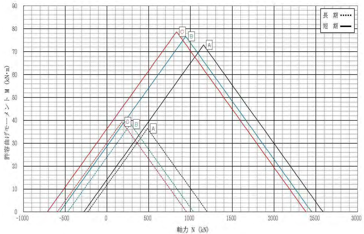
許容曲げモーメント-軸力相関図 \phi 300
