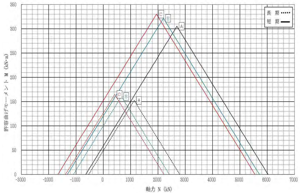
許容曲げモーメント-軸力相関図 \phi 500
