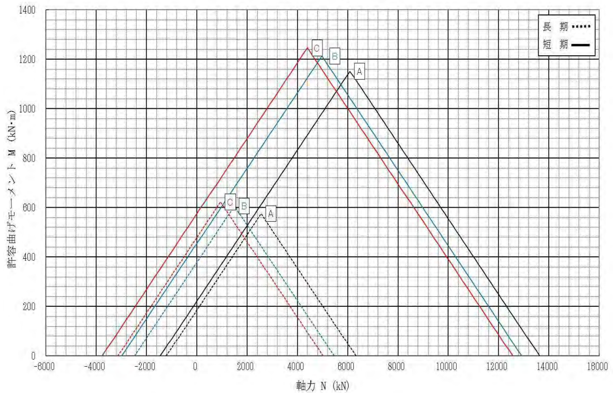
許容曲げモーメント-軸力相関図 \phi 800
