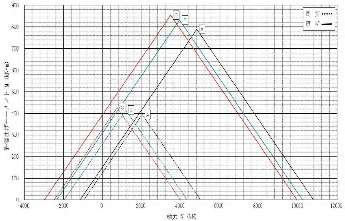
許容曲げモーメント-軸力相関図 \phi 700
