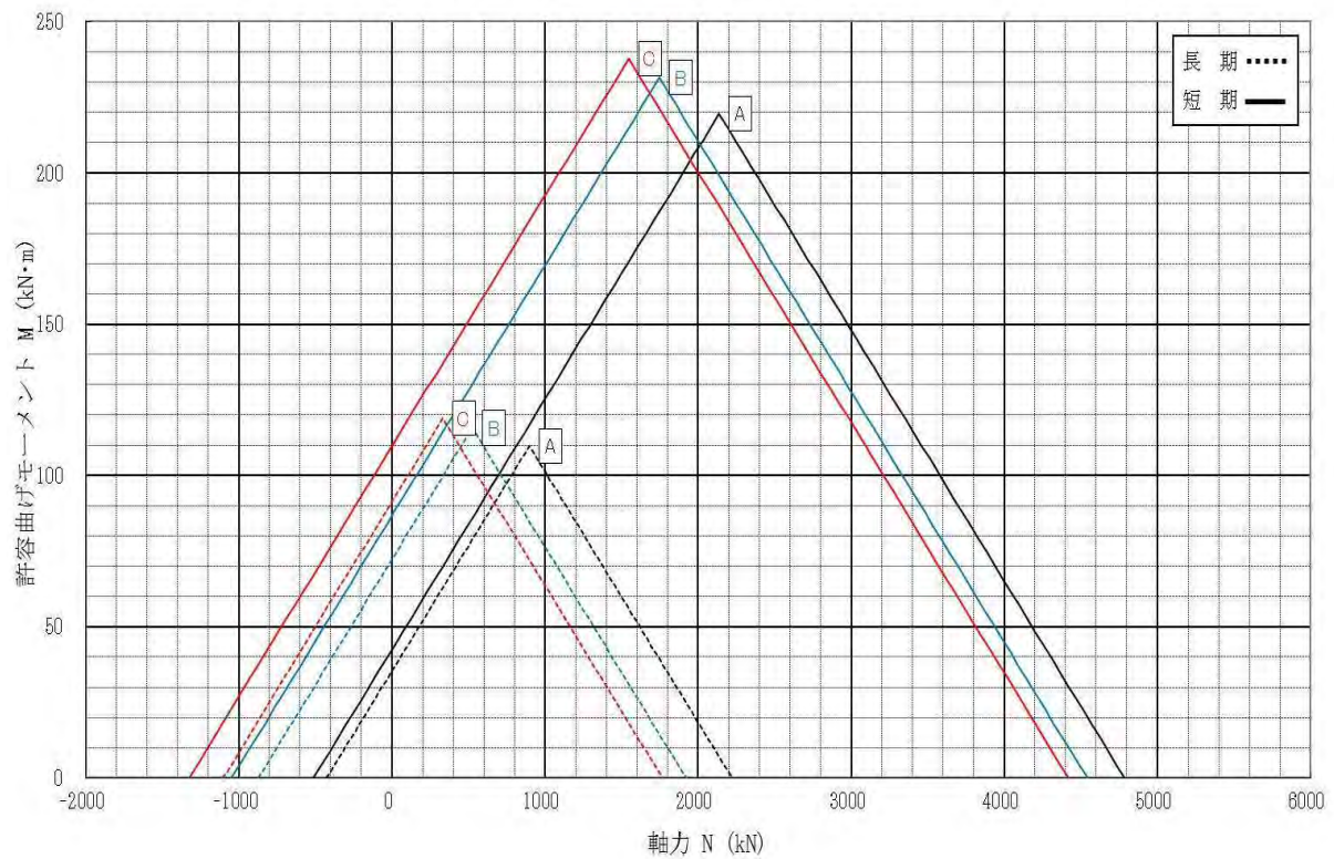
許容曲げモーメント-軸力相関図 \phi 450
