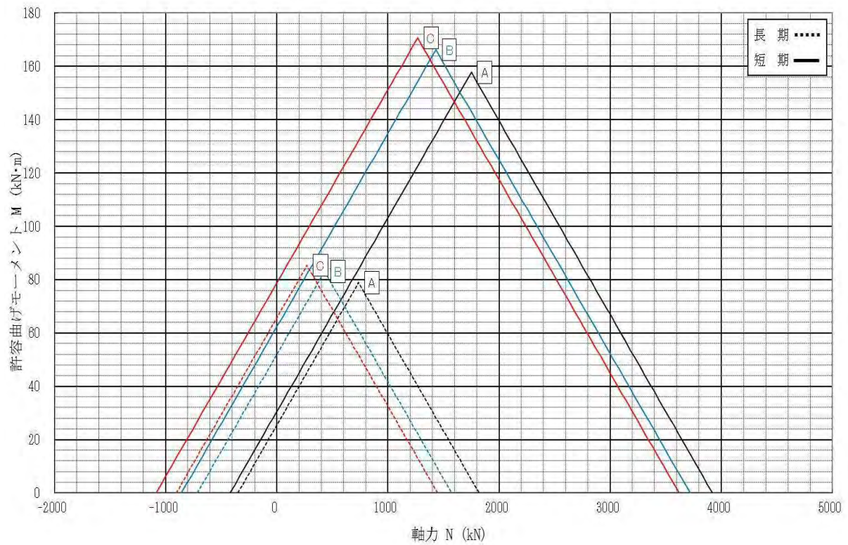
許容曲げモーメント-軸力相関図 \phi 400
