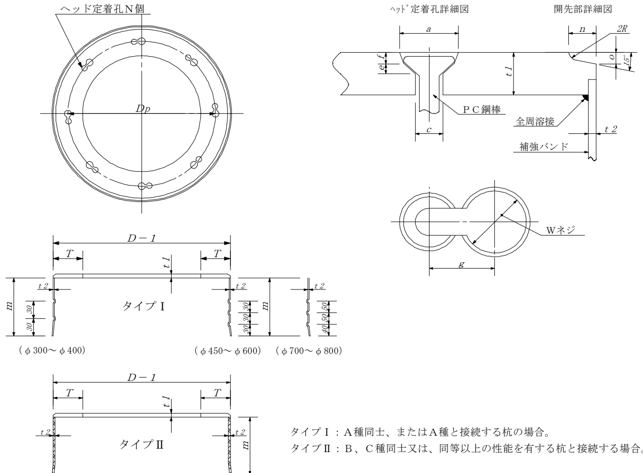
継手部詳細図
