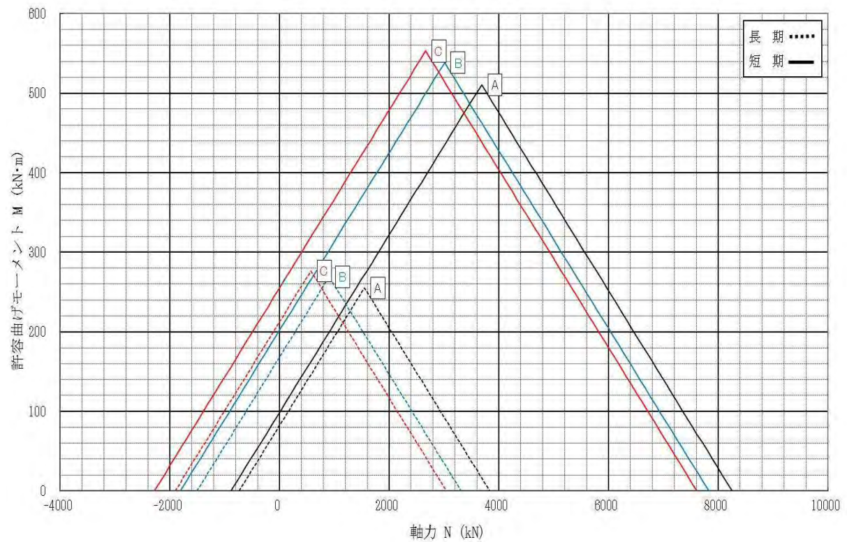
許容曲げモーメント-軸力相関図 \phi 600
