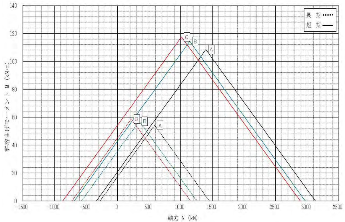
許容曲げモーメント-軸力相関図 \phi 350
