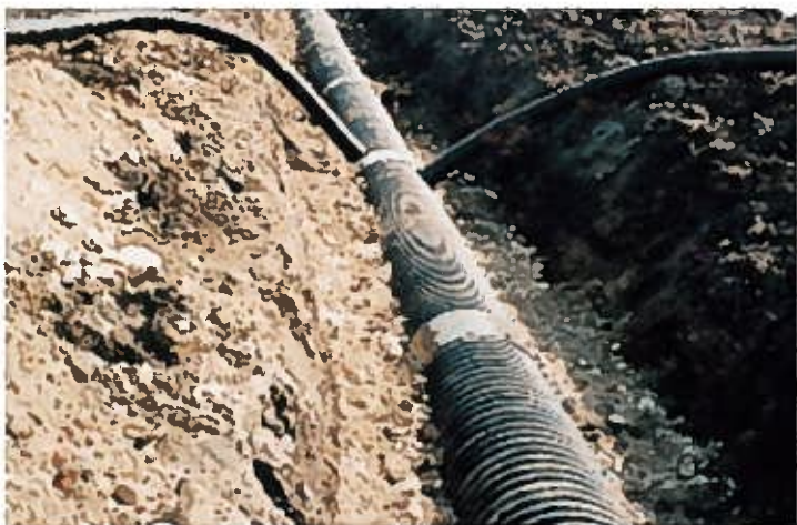
暗渠排水管
